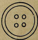
Рис. 97. Правильное решение задачи с пуговицами.
