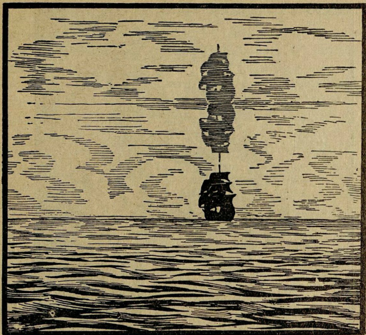
Рис. 105. Мираж на море.
