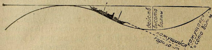
Рис. 38. Почему морские волны с палубы кажутся большей высоты, чем на самом деле?
