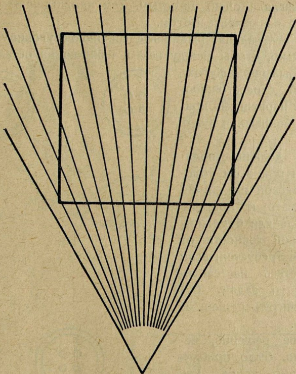
Рис. 98. Квадрат ли начерчен здесь?
