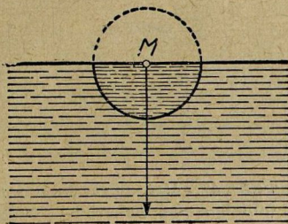
Рис. 44. Частица жидкости на поверхности.
