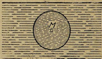
Рис 42. Частица жидкости подвержена действию окружающих частиц.
