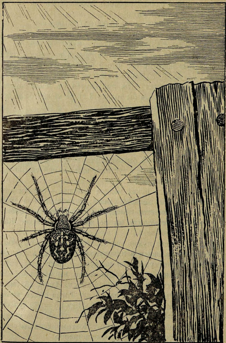
Рис. 4. Можете ли вы рассчитать, сколько должна весить паутинная нить, протянутая от земли до солнца?
