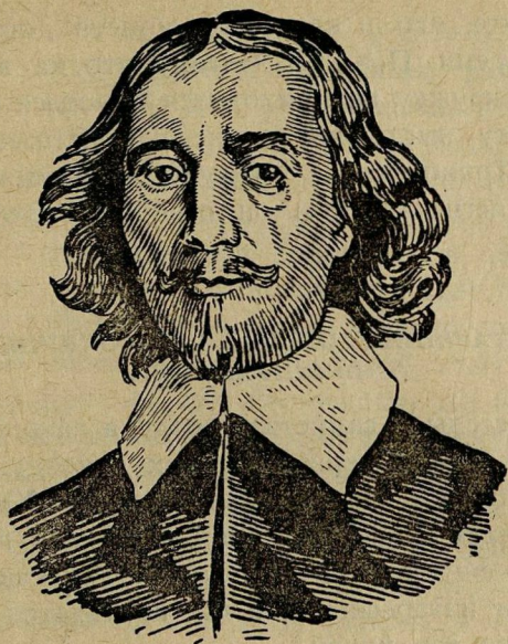
Рис. 63. Отто Герике, изобретатель воздушного насоса.
