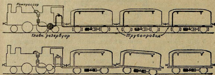
Рис. 59. Устройство воздушного тормоза для остановки поезда. Внизу показано, как действует тормоз в случае разрыва поезда. На обоих рисунках зачернены части, заполненные сжатым воздухом
