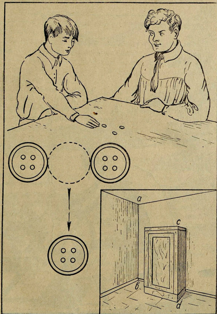
Рис. 96. Опыт с тремя пуговицами. В углу направо — другой обман зрения: линии ab и cd кажутся неодинаковой длины.
