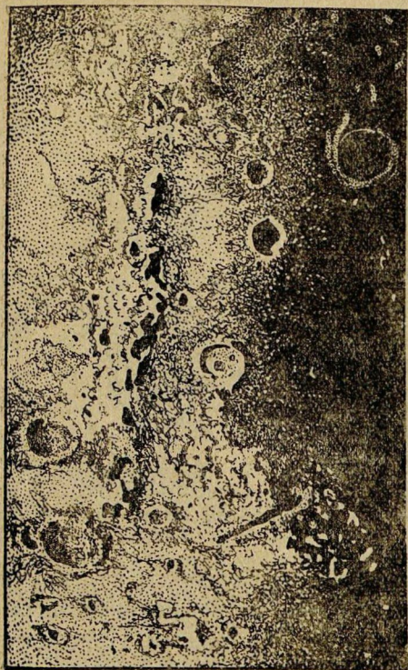
Рис. 91. Что Галилей увидел на поверхности луны.
