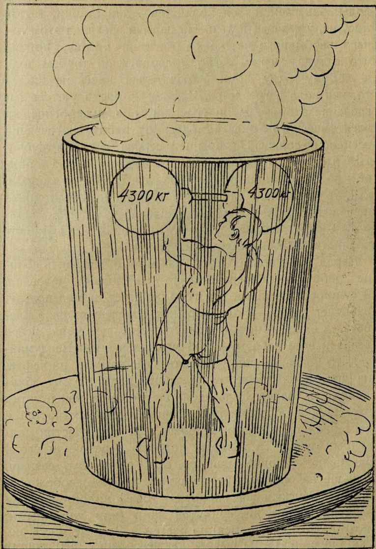
Рис. 77. Невидимый богатырь в стакане чая мог бы поднять груз в 8 600 кг на высоту 1 м.
