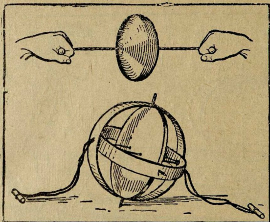
Рис. 29. Почему земной шар раздут у экватора?
