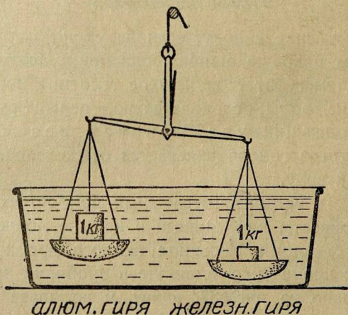
Рис. 36. Задача о весах под водою (ответ).
